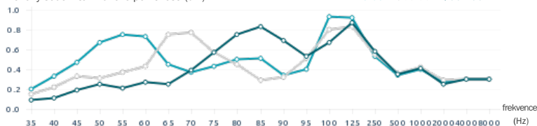
Vážený součinitel zvukové pohltivosti (αw)
